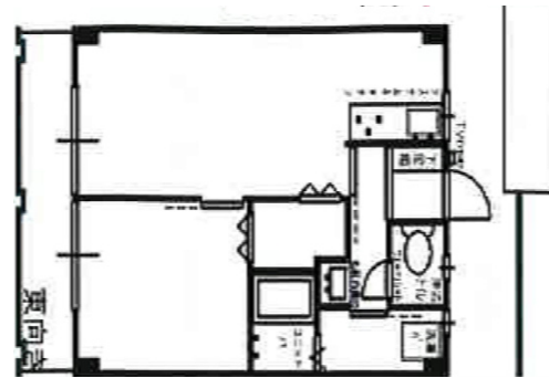
【間取り図】
