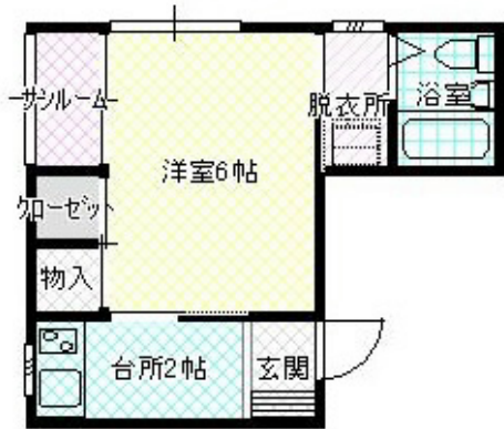
【間取り図】
